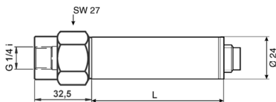
Typ FD 8214 standardní provedení s vnitřním závitem G1/4". D = 45 mm (D = 72mm pro média s teplotou do 150°C, s chladicími žebry)
