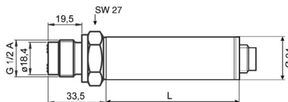
Typ FD8214M membrána v rovině s čelní stranou (svařená s koncem závitu), vnější závit G1/2", snadno sterilizovatelná D = 45 mm (D = 72mm pro média s teplotou do 150°C, s chladicími žebry)
